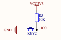
下载按键电路
