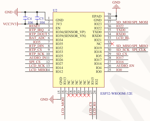
ESP32-WROOM-32E主控电路
