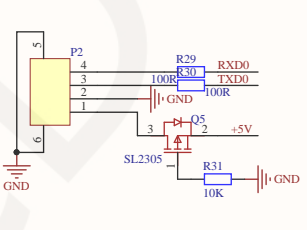
串口模块接口电路
