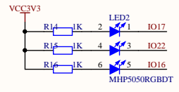
RGB三色灯控制电路 共阳极，低电平点亮 灯
