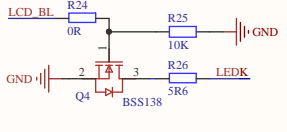
液晶屏背光控制电路
