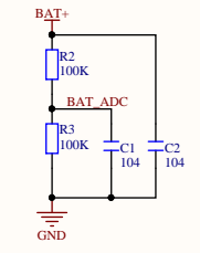
电池电量检测电路
