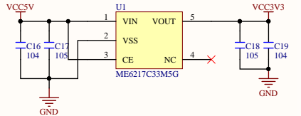
5V转3.3V稳压电路
