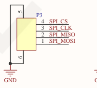
扩展IO以及外设接口电路
