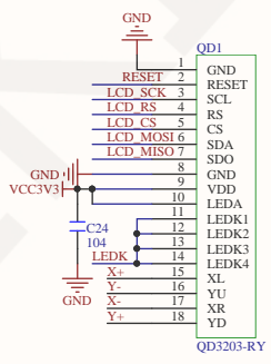
18P液晶屏排线焊接接口
