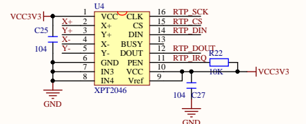
电阻触摸屏控制电路
