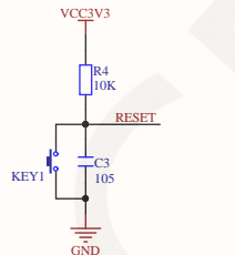
按键复位电路
