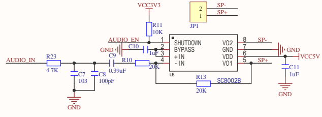
音频功放电路
