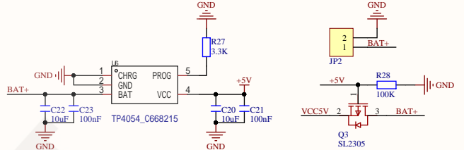
电池充放电管理电路
