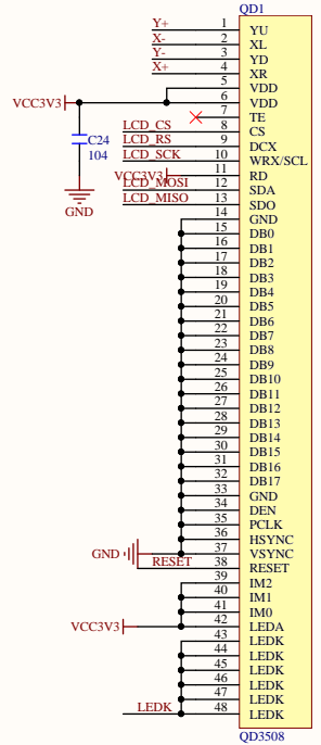
48P液晶屏排线焊接接口
