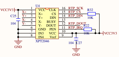
电阻触摸屏控制电路
