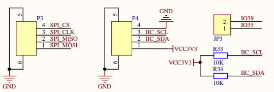
扩展IO以及外设接口电路
