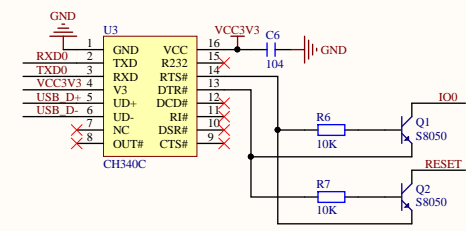
USB转串口以及一键下载电路
