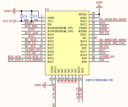
ESP32-WROOM-32E主控电路
