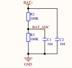
电池电量检测电路
