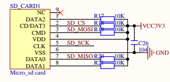
MicroSD卡槽接口电路
