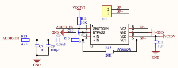
音频功放电路
