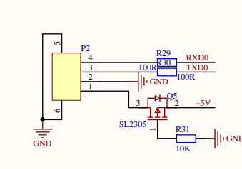
串口模块接口电路
