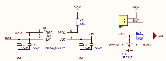
电池充放电管理电路
