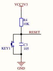
按键复位电路
