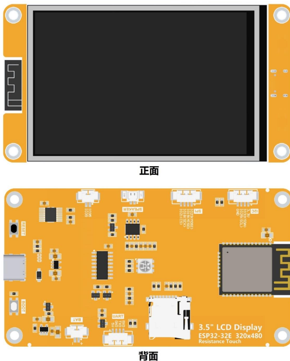
图 1.1 E32R35T 产品图
