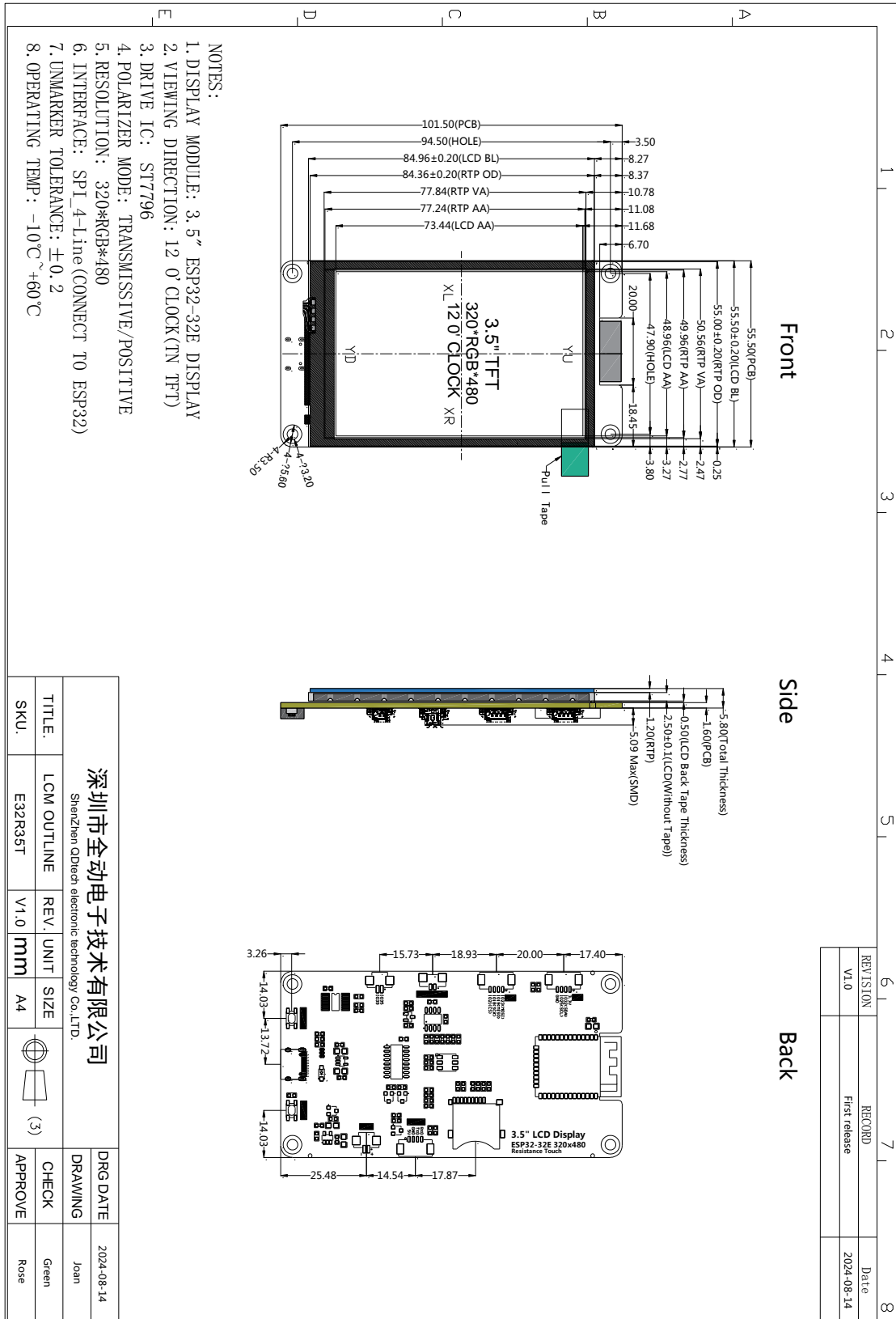
图 5.1 E32R35T 产品尺寸图
